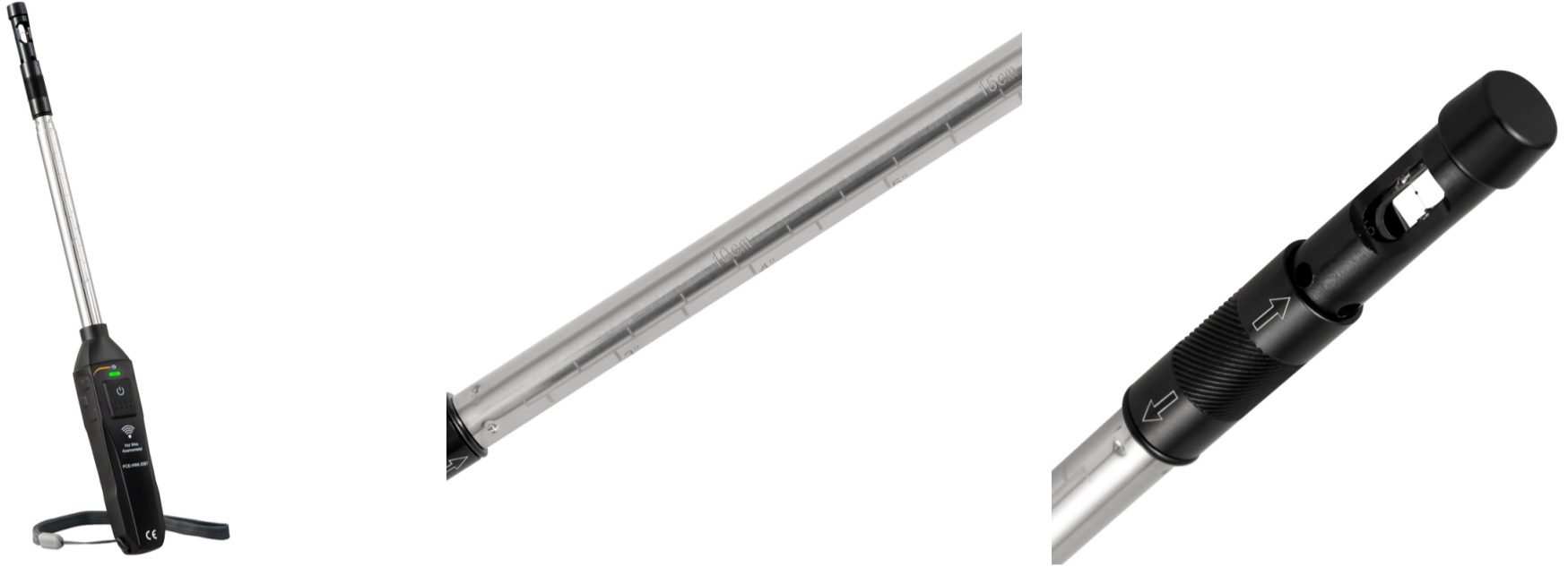
Sıcak Telli Anemometre PCE-HWA 20BT Bluetooth arayüzü / 0 ... 30 m/s ölçüm aralığı / 390 mm uzunluğunda ayarlanabilir teleskopik çubuk / Sıcaklık ve nem ölçümü
