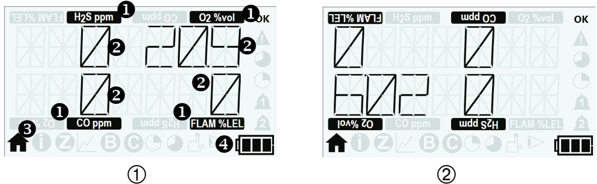
Figura 8: Muestra la pantalla después de un arranque correcto
