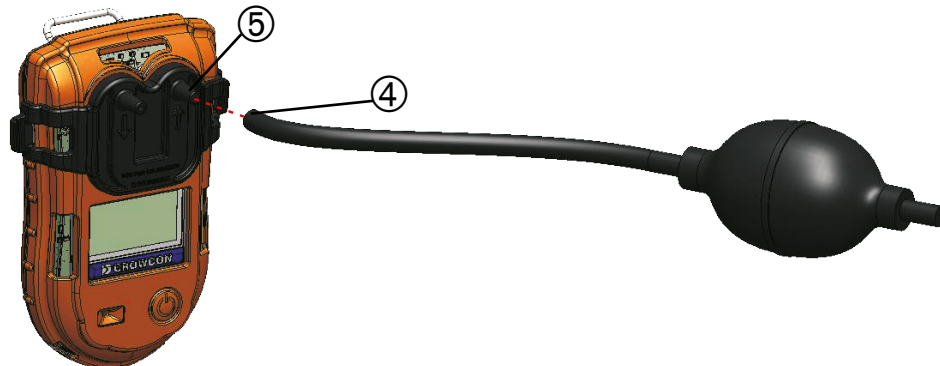
Figura 10: Sujeción del aspirador manual
