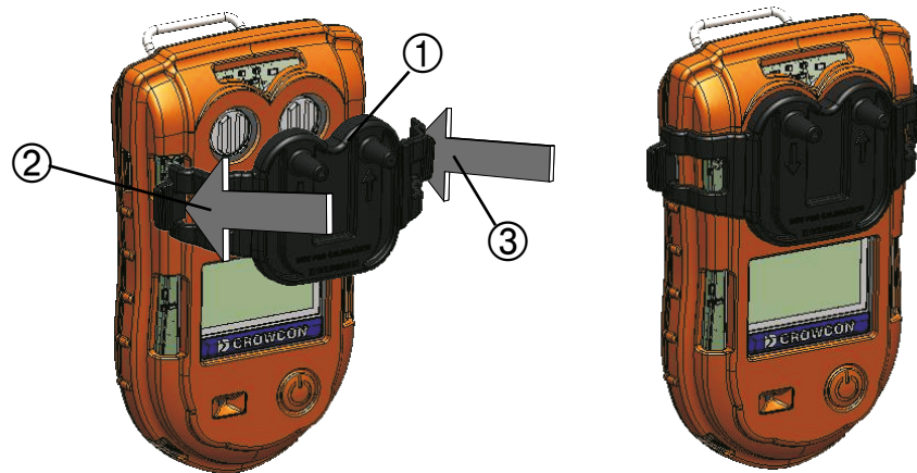
Figura 9: Sujeción de la palanca aspiradora
