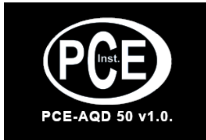
Abb. 3 Boot-Bildschirm
