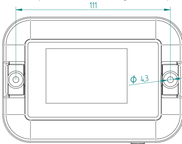
Fig. 37 Drill template
