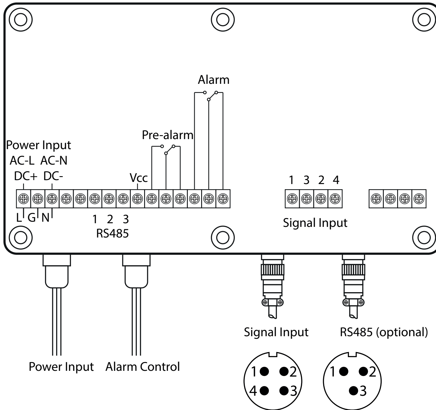
Windwarngerät PCE-WSAC 50
