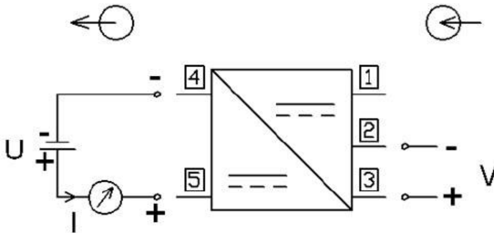
Anschlusskizze vom Signalwandler für 0 - 10 V PCE-P17U
