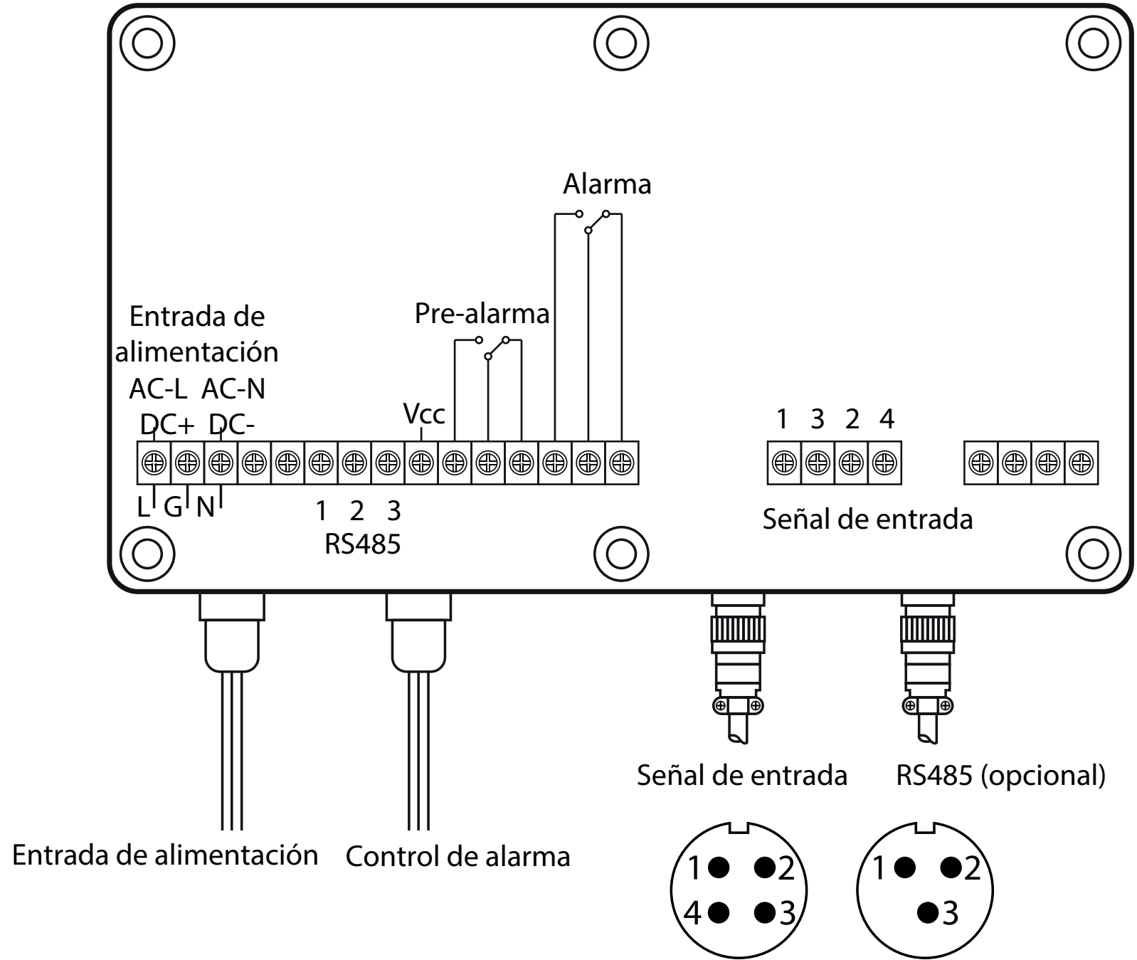
Sistema de alarma de viento PCE-WSAC 50
