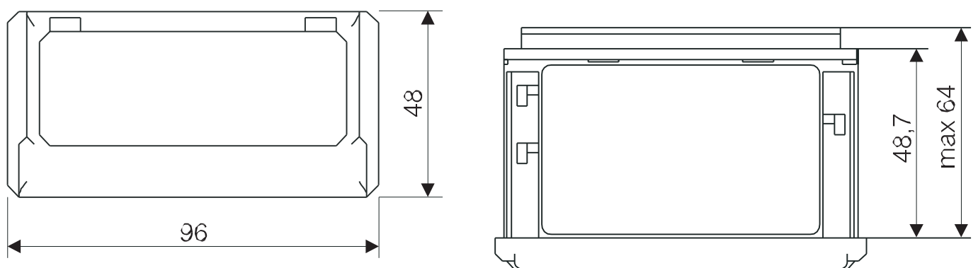
Fig. 2. Dimensiones totales
