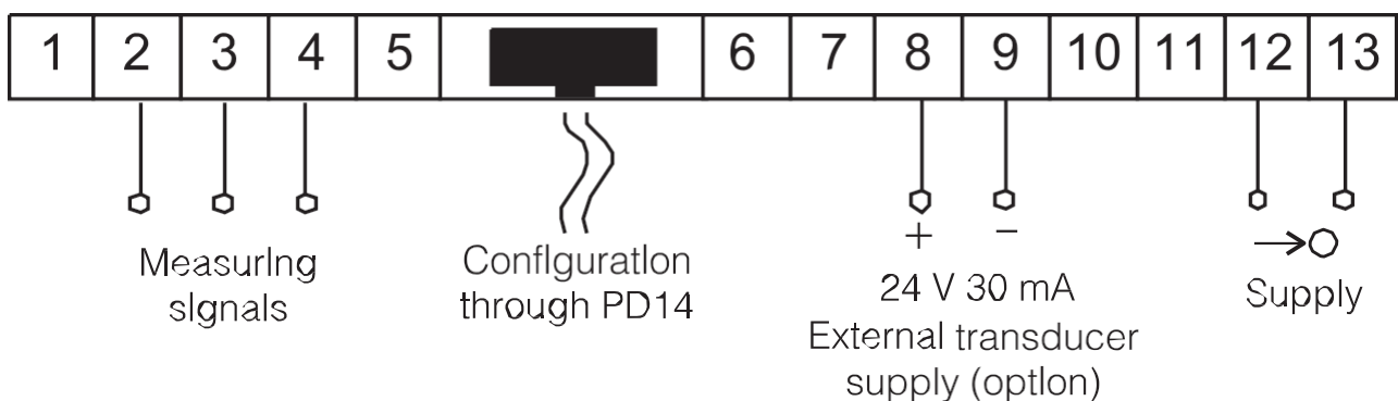
Fig. 4. Conexión eléctrica de los medidores N24T, N25T
